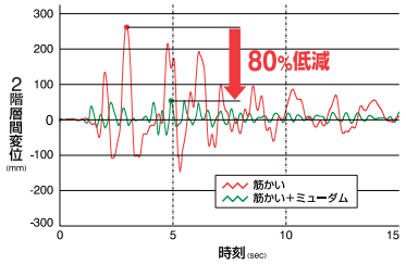
振動台実験による応答変位の時刻歴
