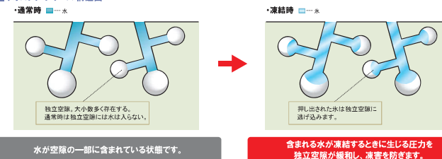
■ネオロック シリーズ構造図
