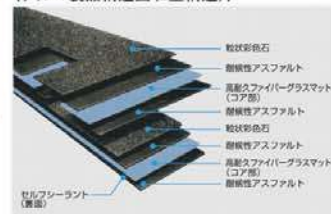
〈アルマ製品構造図(2重構造)〉
